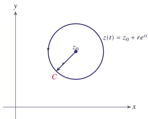
شکل ۱۲.۶۱ دایره C به مرکز z_0 و شعاع r
