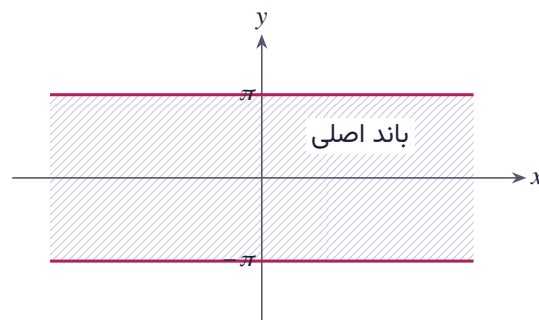
شکل ۱۰.۴۱ باند اصلی تابع نمایی: -\pi < y \leq \pi
