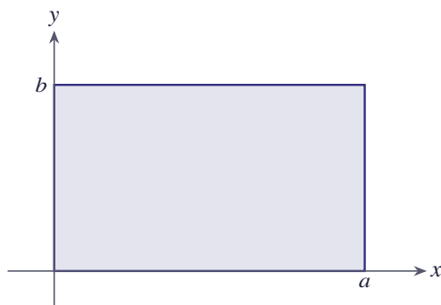
شکل ۶.۲۵ ناحیه مستطیلی 0 \leq x \leq a, 0 \leq y \leq b
