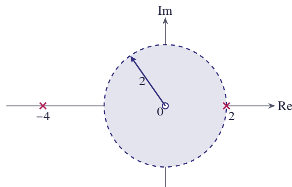
شکل ۱۳.۷۲ قطب‌های z = 2 و z = -4 ؛ دایره همگرایی حول مبدأ شعاع ۲ دارد
