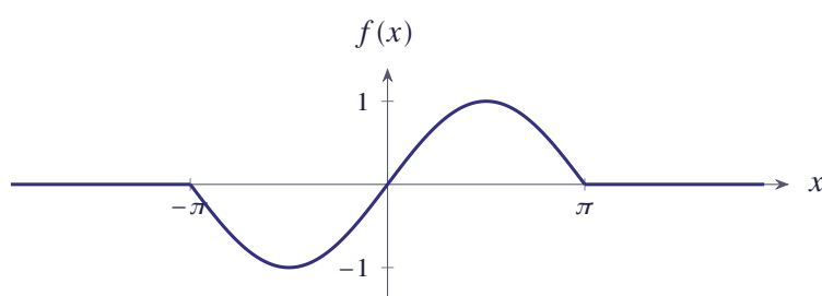
شکل ۳.۵ تابع f(x) = \sin x برای |x| \leq \pi و صفر در بیرون
