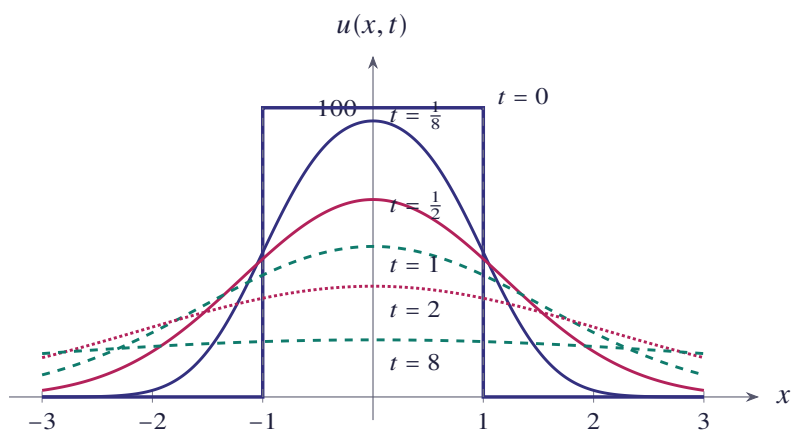
شکل ۵.۳ توزیع دما u(x, t) در لحظه‌های t = 0, \frac{1}{8}, \frac{1}{2}, 1, 2 و ۸ برای پالس اولیه U_0 = 100 و c = 1
