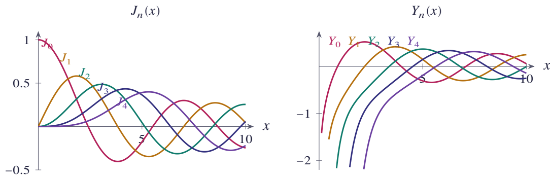
شکل ۶.۵ توابع بسل نوع اول J_0, \dots, J_4 و نوع دوم Y_0, \dots, Y_4 برای 0 < x \leq 10
