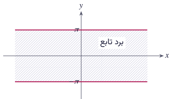
شکل ۱۰.۴ برد تابع لگاریتم: نوار -\pi < \operatorname{Im} w \leq \pi
