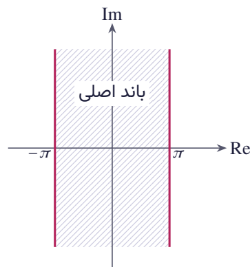
شکل ۱۰.۲ باند اصلی توابع \cos z و \sin z : -\pi < x \leq \pi
