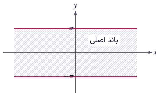
شکل ۱۰.۱ باند اصلی تابع نمایی: -\pi < y \leq \pi
