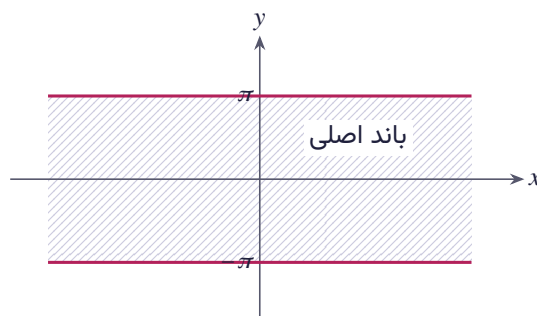
شکل ۱۰.۳ باند اصلی توابع هذلولی‌گون: -\pi < y \leq \pi
