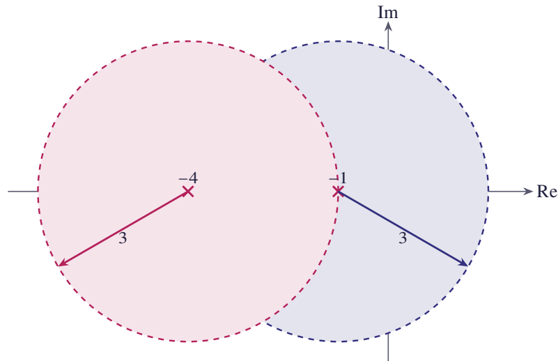
شکل ۱۳.۵ قطب‌های z = -1 و z = -4 تابع f(z) = \frac{z}{(z+1)(z+4)^3}
