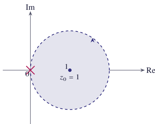
شکل ۱۳.۴ ناحیه همگرایی سری حول z_0 = 1 دایره‌ای به شعاع ۱ است (تا قطب z = 0 )
