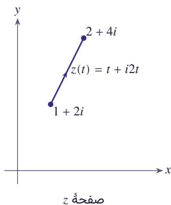
شکل ۱۲.۳ مسیر z(t) = t + i2t , 1 \leq t \leq 2
