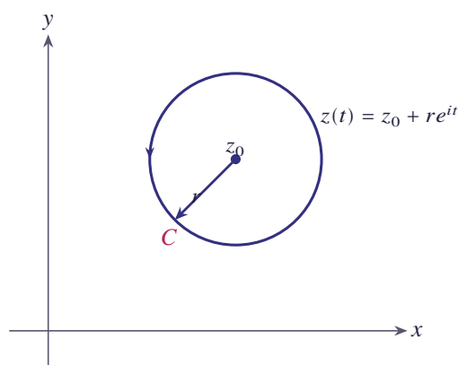
شکل ۱۲.۱۳ دایره C به مرکز z_0 و شعاع r
