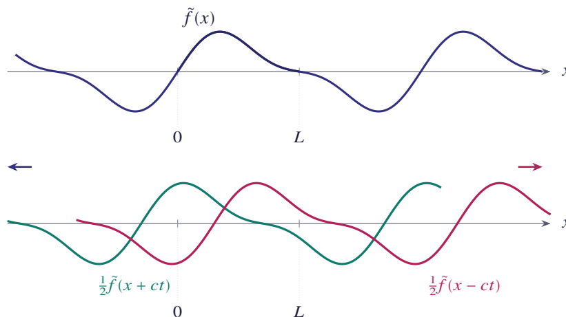
شکل ۴.۱۹ ادامه فرد و متناوب \tilde{f}(x) و دو موج \frac{1}{2}\tilde{f}(x+ct) و \frac{1}{2}\tilde{f}(x-ct) که در دو جهت مخالف حرکت می‌کنند
