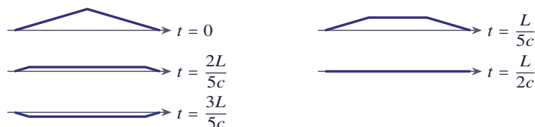
شکل ۴.۲۰ جواب مثال برای t = 0, \frac{L}{5c}, \frac{2L}{5c}, \frac{3L}{5c}, \frac{L}{2c} ؛ در t = \frac{L}{2c} شکل تار صاف است
