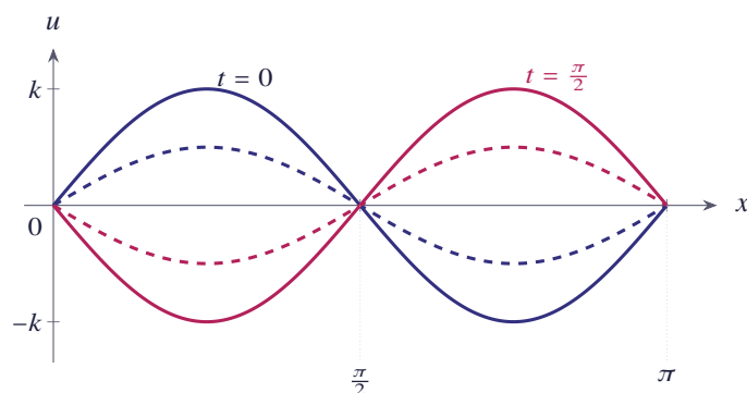
شکل ۴.۱۶ مود دوم ارتعاش تار: u(x, t) = k \sin 2x \cos 2t در لحظه‌های مختلف
