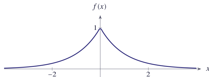
شکل ۳.۱۳ تابع f(x) = e^{-|x|}
