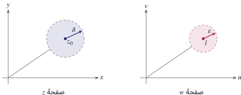
شکل ۹.۳۷ تعریف حد: دایره \delta -همسایگی z_0 در صفحه z و دایره \epsilon -همسایگی l در صفحه w
