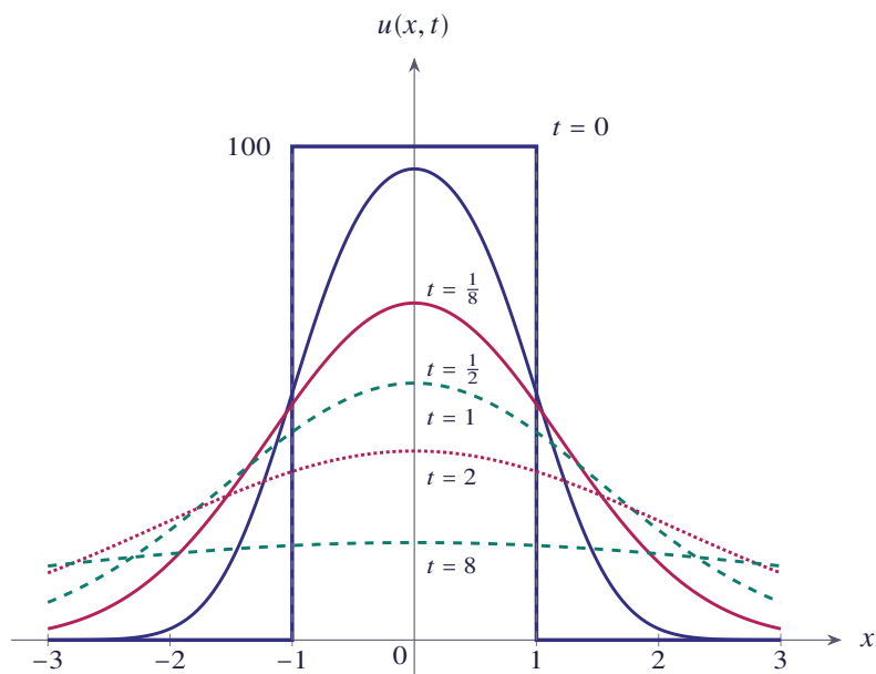
شکل ۵.۲۳ توزیع دما u(x, t) در لحظه‌های t = 0, \frac{1}{8}, \frac{1}{2}, 1, 2 و ۸ برای پالس اولیه U_0 = 100 و c = 1
