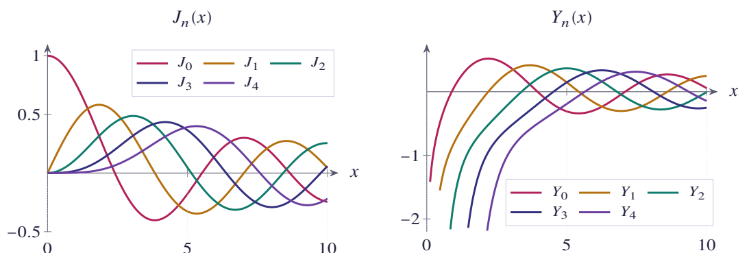
شکل ۶.۲۸ توابع بسل نوع اول J_0, \dots, J_4 و نوع دوم Y_0, \dots, Y_4 برای 0 < x \leq 10
