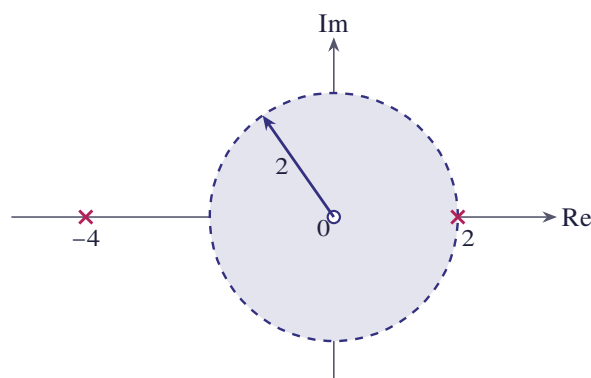
شکل ۱۳.۷۲ قطب‌های z = -4 و z = 2 ؛ دایره همگرایی حول مبدأ شعاع ۲ دارد
