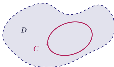
شکل ۱۲.۵۹ مسیر ساده بسته C در ناحیه همبند ساده D
