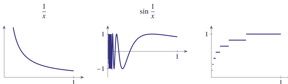
شکل ۱.۸ توابعی که شرایط دریشه را ندارند: \frac{1}{x} (نامحدود)، \sin \frac{1}{x} (بی‌نهایت ماکزیمم و مینیمم) و تابع پله‌ای با بی‌نهایت پله
