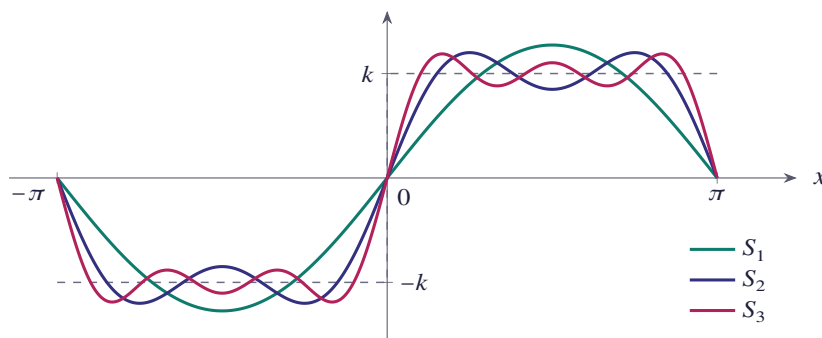
شکل ۱.۴ مجموع‌های جزئی S_1 ، S_2 و S_3 سری فوریه موج مربعی (خط چین خود موج مربعی است)
