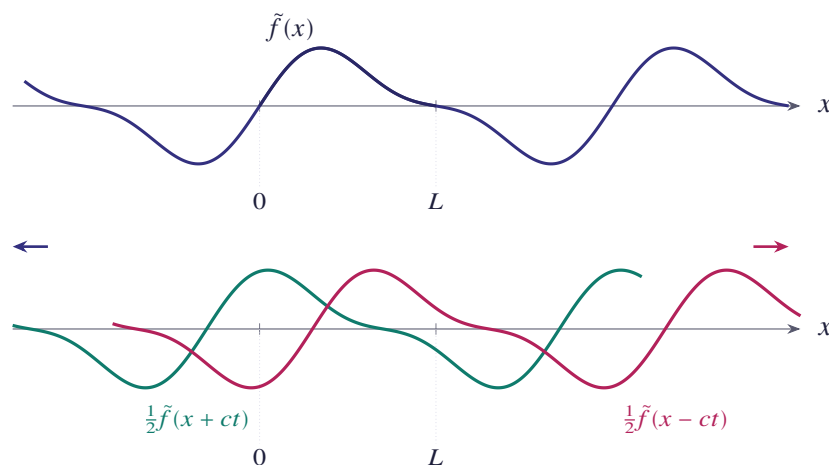
شکل ۴.۵ ادامه فرد و متناوب \tilde{f}(x) و دو موج \frac{1}{2}\tilde{f}(x+ct) و \frac{1}{2}\tilde{f}(x-ct) که در دو جهت مخالف حرکت می‌کنند
