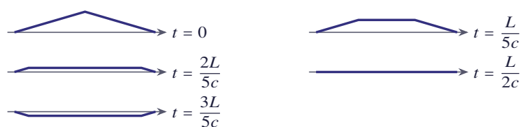
شکل ۴.۶ جواب مثال برای t = 0 ، \frac{L}{5c} ، \frac{2L}{5c} ، \frac{L}{2c} و \frac{3L}{5c} ؛ در t = \frac{L}{2c} شکل تار صاف است
