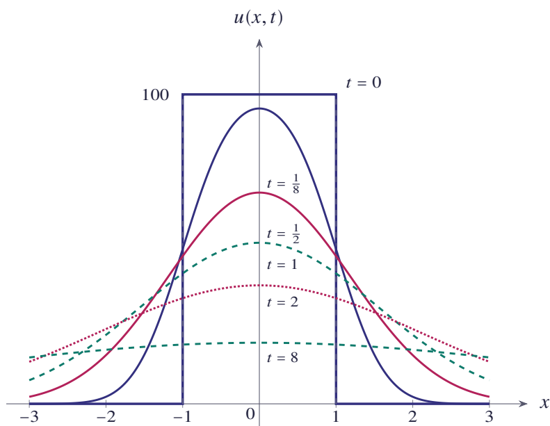
شکل ۵.۳ توزیع دما u(x, t) در لحظه‌های t = 0, \frac{1}{8}, \frac{1}{2}, 1, 2, 8 برای پالس اولیه U_0 = 100 و c = 1
