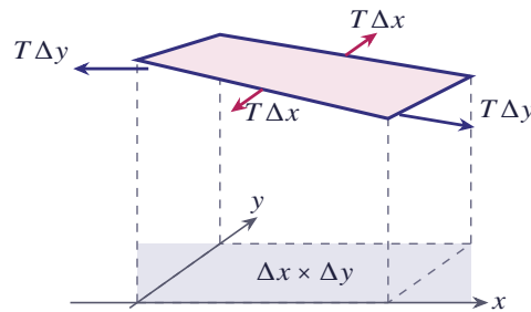
شکل ۶.۱ المان \Delta x \times \Delta y از غشاء مرتعش و نیروهای کششی T\Delta x و T\Delta y وارد بر آن
