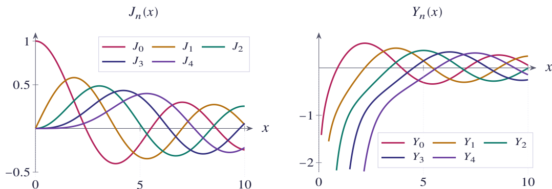
شکل ۶.۵ توابع بسل نوع اول J_0, \dots, J_4 و نوع دوم Y_0, \dots, Y_4 برای 0 < x \leq 10
