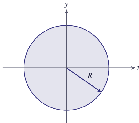
شکل ۶.۴ غشاء دایره‌ای به شعاع R
