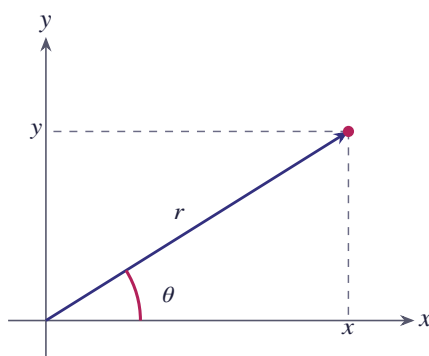
شکل ۶.۳ مختصات قطبی: x = r \cos \theta , y = r \sin \theta
