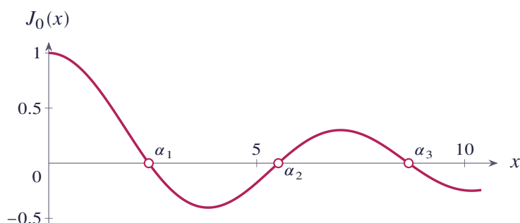
شکل ۶.۶ تابع J_0(x) و ریشه‌های آن \alpha_1, \alpha_2, \alpha_3
