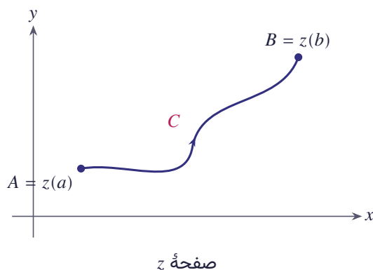
شکل ۱۲.۲ مسیر C با جهت از A = z(a) به B = z(b)
