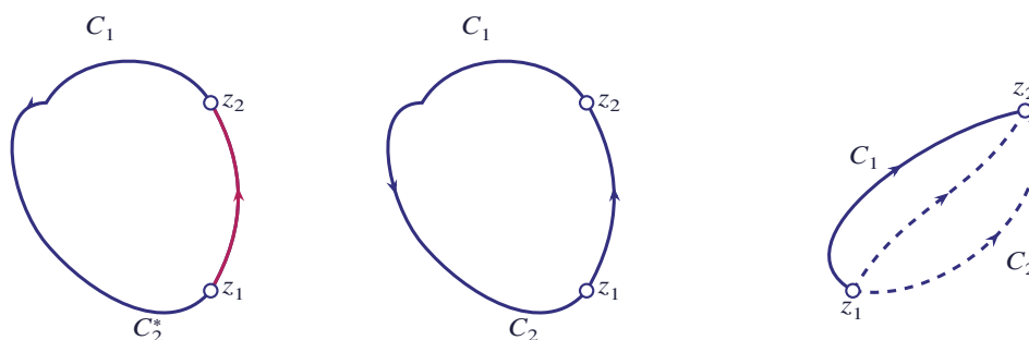
شکل ۱۲.۱۲ مسیرهای C_1 ، C_2 و C_2^* (مسیر C_2 با جهت معکوس) میان z_1 و z_2
