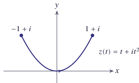
شکل ۱۲.۶ مسیر z(t) = t + it^2 ، -1 \leq t \leq 1 از -1 + i تا 1 + i
