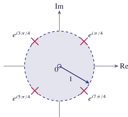
شکل ۱۳.۲ چهار قطب z^4 + 1 = 0 روی دایره واحد؛ شعاع همگرایی سری حول مبدأ برابر ۱ است
