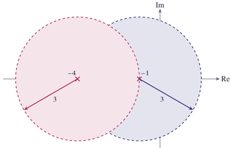
شکل ۱۳.۵ قطب‌های z = -4 و z = -1 تابع f(z) = \frac{z}{(z+1)(z+4)^3}
