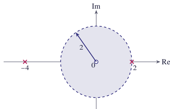
شکل ۱۳.۳ قطب‌های z = 2 و z = -4 ؛ دایره همگرایی حول مبدأ شعاع ۲ دارد
