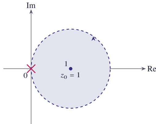
شکل ۱۳.۴ ناحیه همگرایی سری حول z_0 = 1 دایره‌ای به شعاع ۱ است (تا قطب z = 0 )
