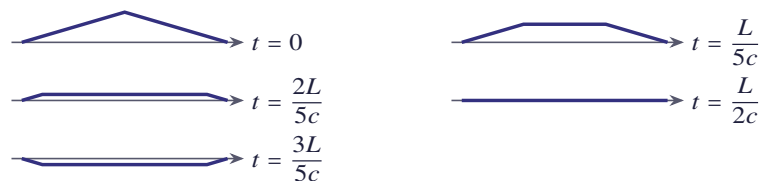
شکل ۴.۲۰ جواب مثال برای t = 0 ، \frac{L}{5c} ، \frac{2L}{5c} ، \frac{L}{2c} و \frac{3L}{5c} در شکل تار صاف است
