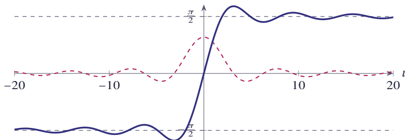
شکل ۳.۱۱ تابع \text{Si}(u) (خط ممتد) و تابع \frac{\sin u}{u} (خط چین)
