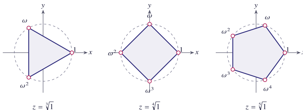
شکل ۸.۳۴ ریشه‌های z = \sqrt[n]{1} , z = \sqrt[n]{1} و z = \sqrt[n]{1} روی دایره واحد
