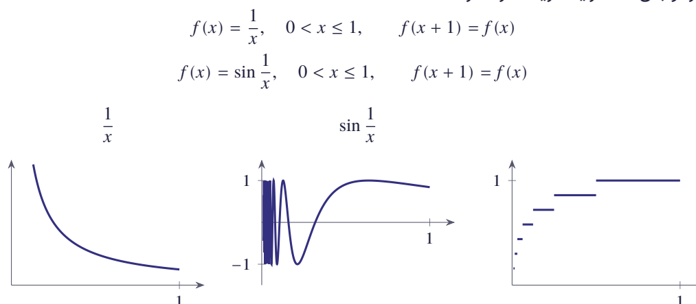
شکل ۱.۸ توابعی که شرایط دریشه را ندارند: \frac{1}{x} (نامحدود)، \sin \frac{1}{x} (بی‌نهایت ماکزیمم و مینیمم) و تابع پله‌ای با بی‌نهایت پله
