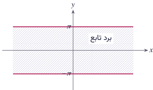
شکل ۱۰.۴۴ برد تابع لگاریتم: -\pi < \text{Im } w \leq \pi
