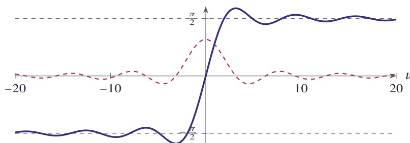
شکل ۳.۲ تابع Si(u) (خط ممتد) و تابع \frac{\sin u}{u} (خط چین)
