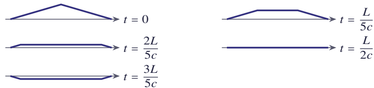
شکل ۴.۶ جواب مثال برای t = 0 ، \frac{L}{5c} ، \frac{2L}{5c} ، \frac{L}{2c} و \frac{3L}{5c} ؛ در t = \frac{L}{2c} شکل تار صاف است
