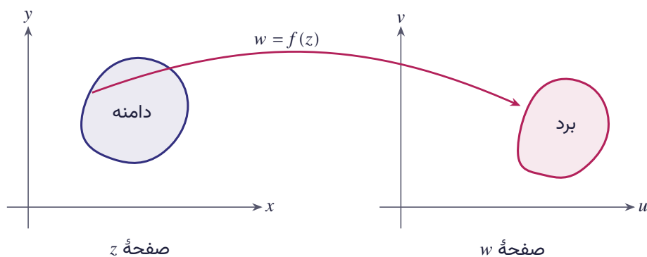
شکل ۹.۱ تابع مختلط w = f(z) نقاط دامنه در صفحه z را به نقاط برد در صفحه w می‌نگارد
