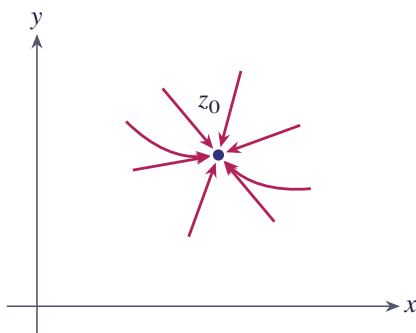
شکل ۹.۵ نزدیک شدن به نقطه z_0 از تمام جهات
