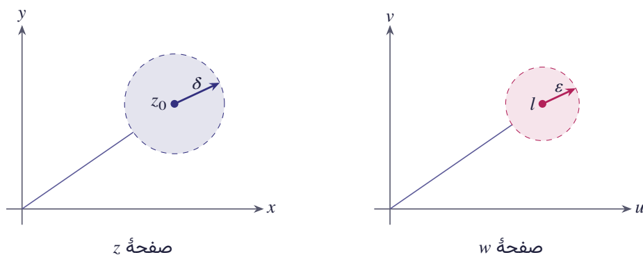
شکل ۹.۳ تعریف حد: دایره \delta -همسایگی z_0 در صفحه z و دایره \epsilon -همسایگی l در صفحه w
