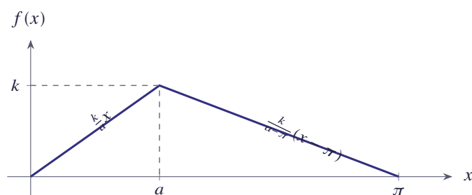
شکل ۴.۱۷ توزیع اولیه مثلثی f(x) با قله k در x = a
