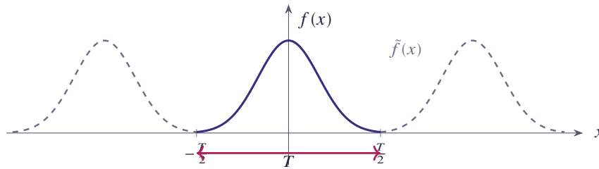
شکل ۳.۱۰ تابع غیرتناوبی f(x) و ادامه متناوب آن \tilde{f}(x) با دوره تناوب T
