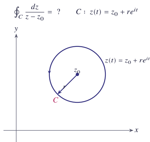
شکل ۱۲.۶۱ دایره C به مرکز z_0 و شعاع r
