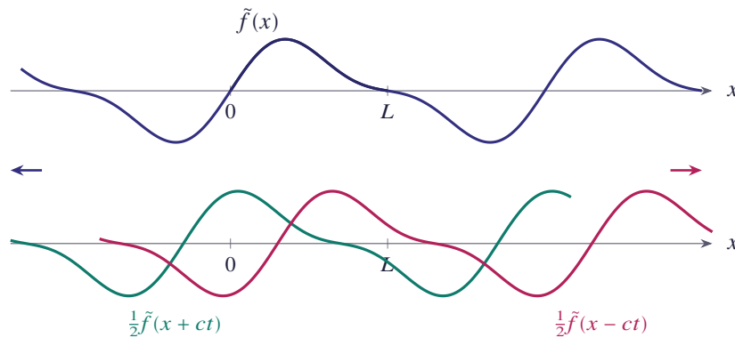
شکل ۴.۱۹ ادامه فرد و متناوب \tilde{f}(x) و دو موج \frac{1}{2}\tilde{f}(x + ct) و \frac{1}{2}\tilde{f}(x - ct) که در دو جهت مخالف حرکت می‌کنند
