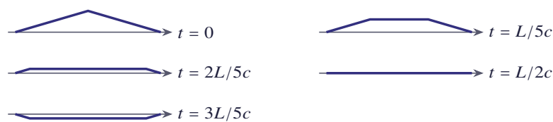
شکل ۴.۲۰ جواب مثال برای t = 0, L/5c, 2L/5c, L/2c, 3L/5c در t = L/2c شکل تار صاف است
