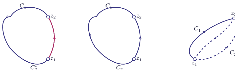
شکل ۱۲.۶۰ مسیره‌های C_1 ، C_2 و C_2^* (مسیر C_2 با جهت معکوس) میان z_1 و z_2
