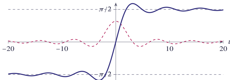
شکل ۳.۱۱ تابع \text{Si}(u) (خط ممتد) و تابع \sin u/u (خط چین)
