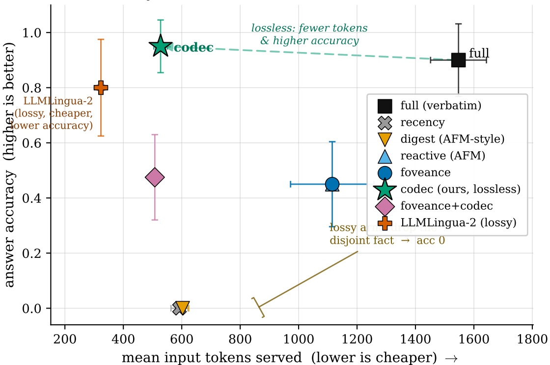
Accuracy-token frontier: the lossless codec dominates
