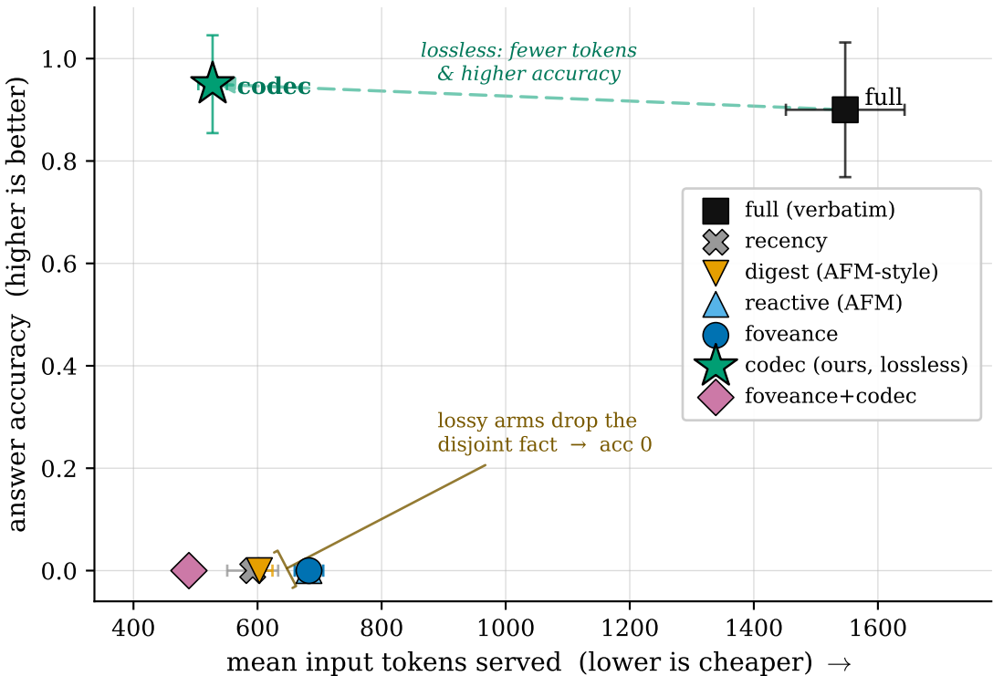
Accuracy-token frontier: the lossless codec dominates
