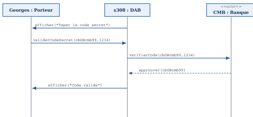
Scenario nominal du cas d'utilisation "S'authentifier"
