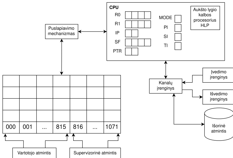
1 pav. Realios mašinos schema
