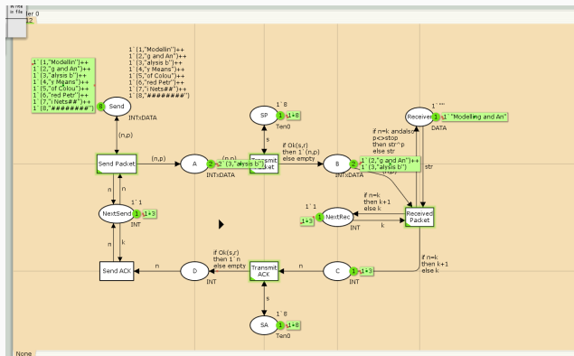
Рис. 5: Запуск модели простого протокола передачи данных
