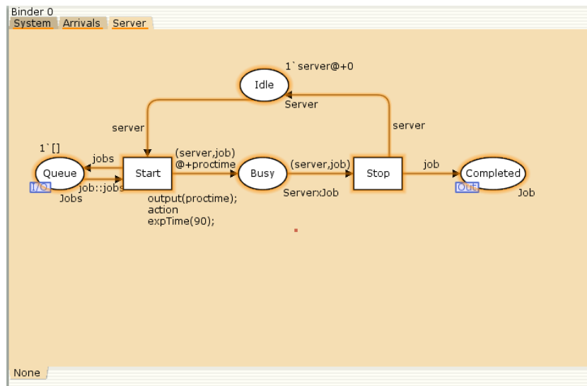
Рис. 3.7: Параметры элементов обработчика заявок системы
