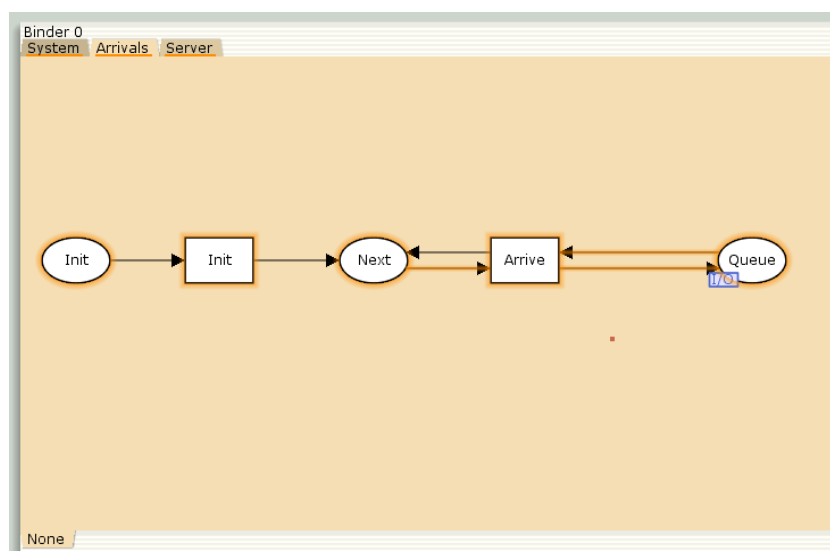
Рис. 3.2: Граф генератора заявок системы
