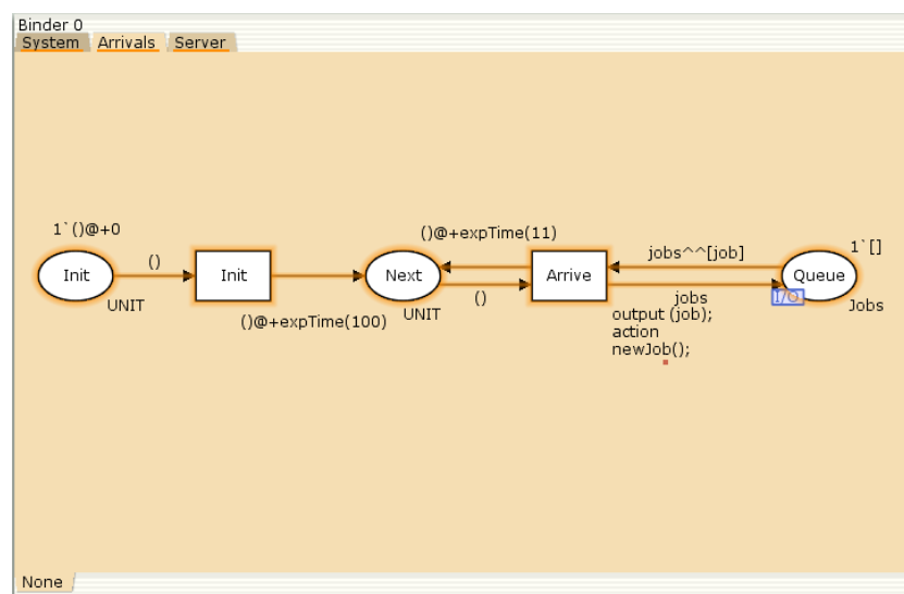
Рис. 3.6: Параметры элементов генератора заявок системы
