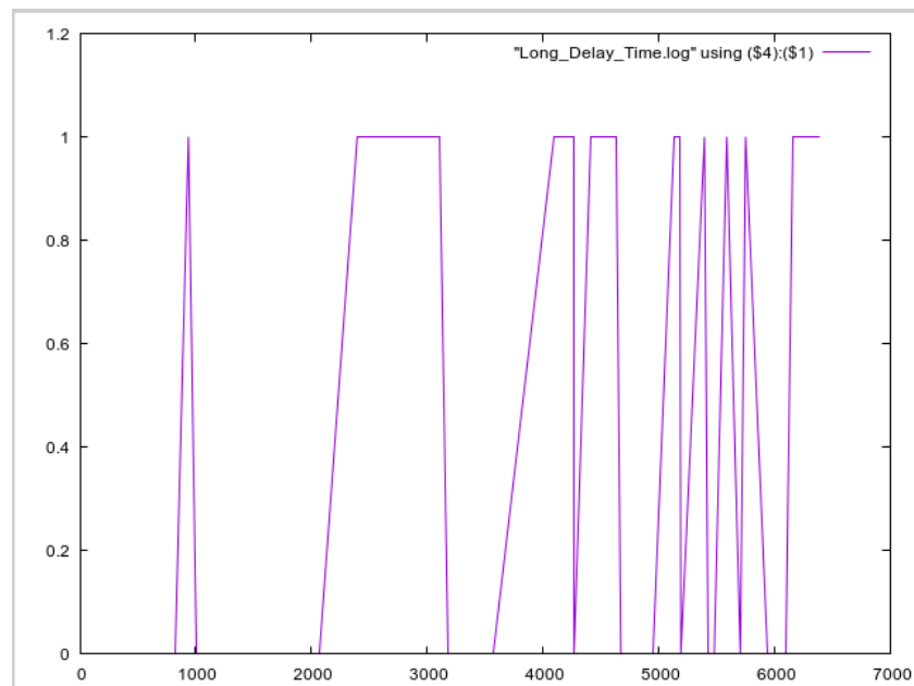
Рис. 3.18: Периоды времени, когда значения задержки в очереди превышали заданное значение
