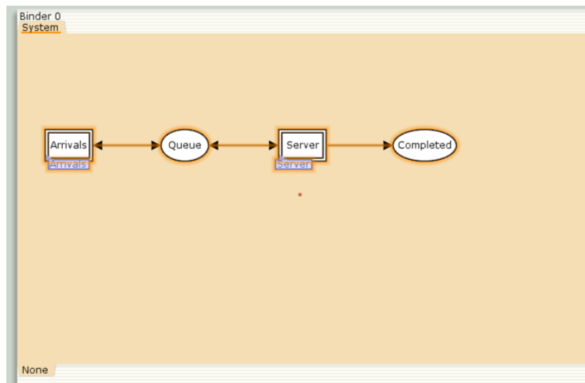
Рис. 3.1: Граф сети системы обработки заявок в очереди
