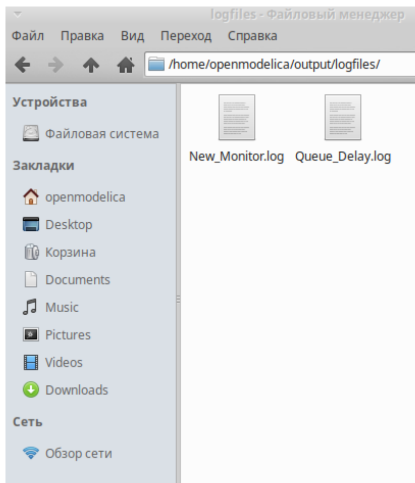
Рис. 3.13: Файл Queue_Delay.log
