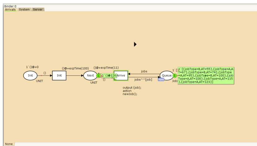
Рис. 3.8: Arrivals
