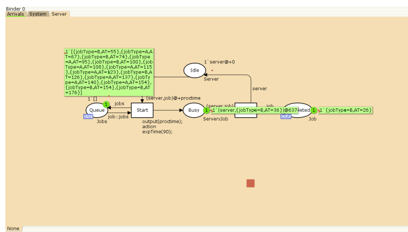
Рис. 3.10: Server
