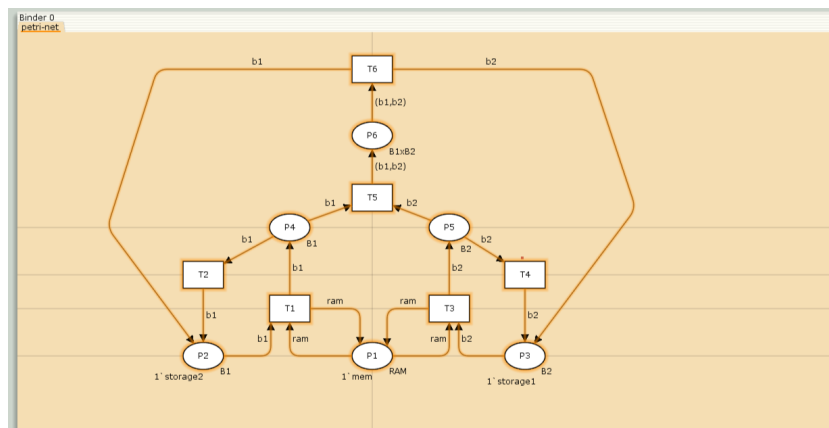
Рис. 2.3: Модель задачи в CPN Tools
