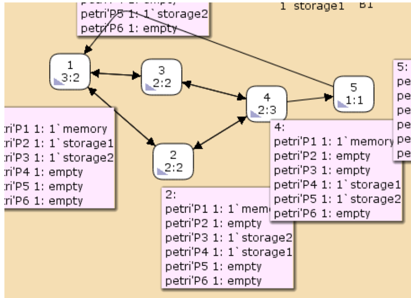
Рис. 2.7: Граф пространства состояний
