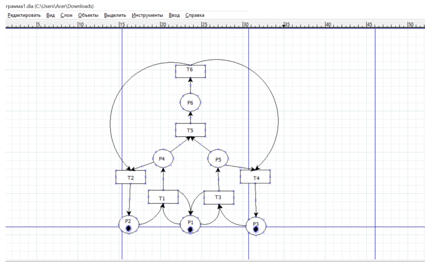
Рис. 2.1: Сеть для выполнения домашнего задания
