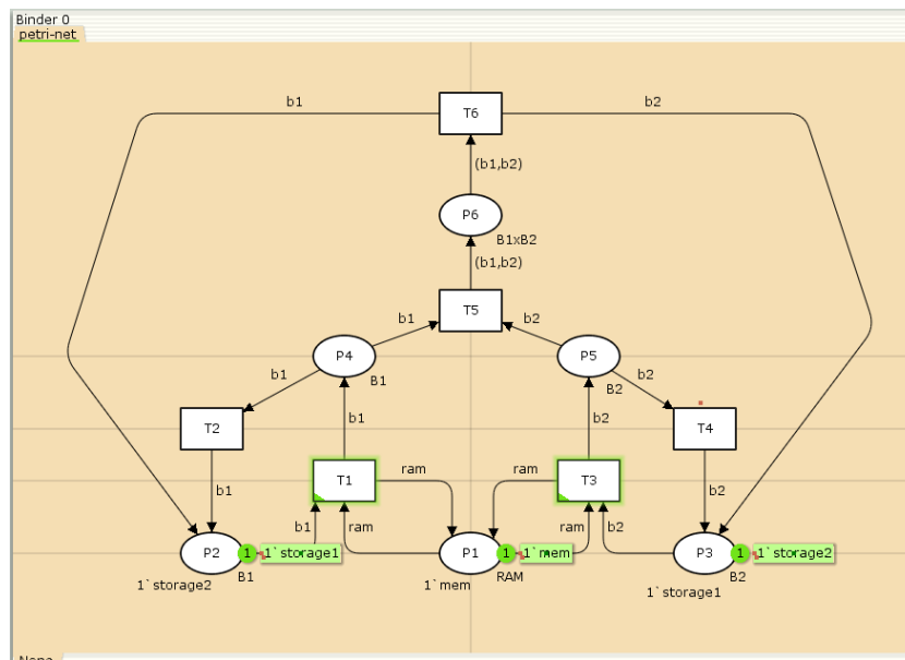
Рис. 2.5: Модель задачи в CPN Tools
