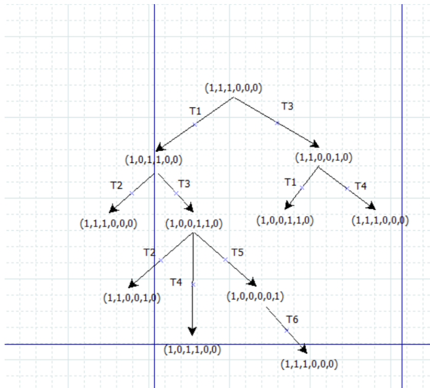
Рис. 2.2: Дерево достижимости
