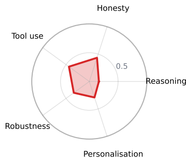
sft template
