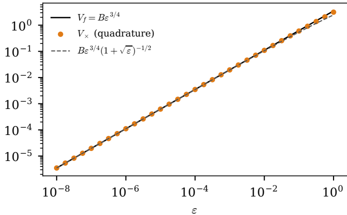
(b) sublevel area, slope 3/4
