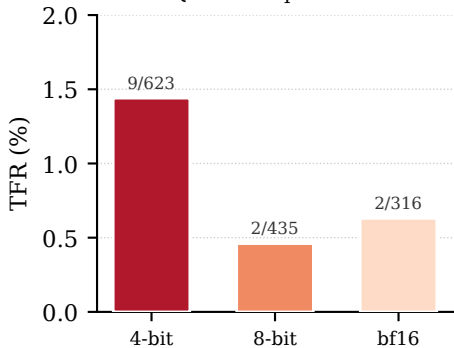
Qwen3-8B precision
