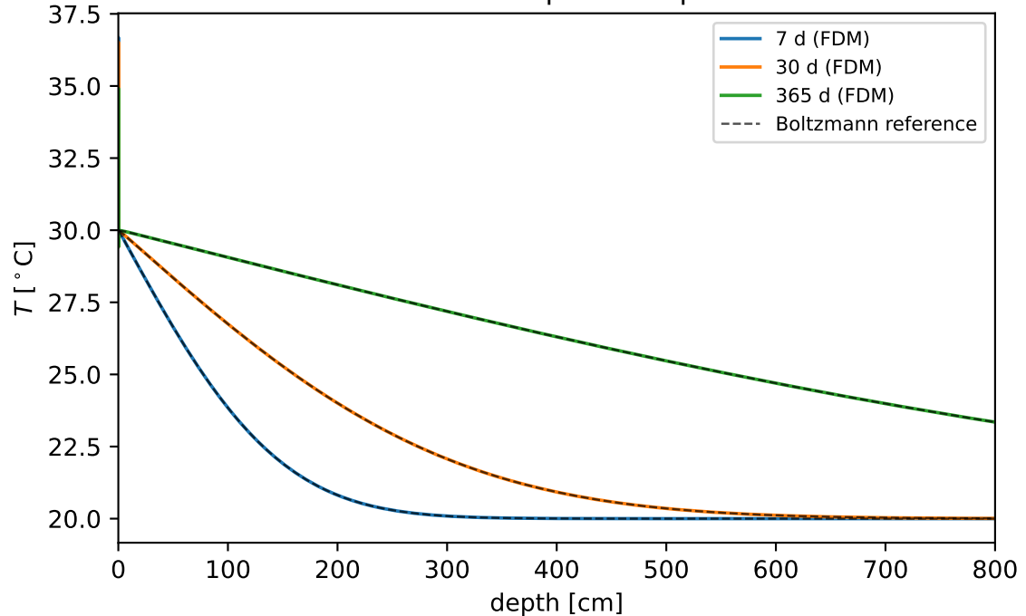
EN 15026: temperature profiles
