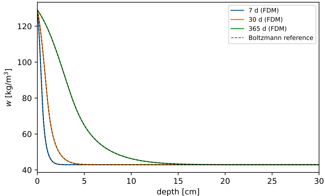
EN 15026: moisture profiles
