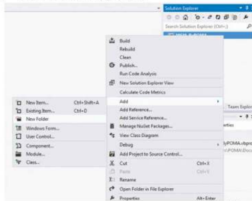
Gambar 5.8 Menambahkan Folder
