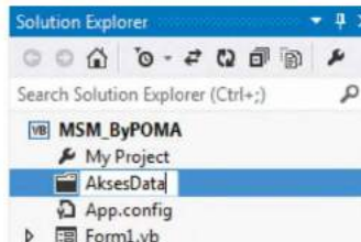
Gambar 5.8 Menambahkan Folder
