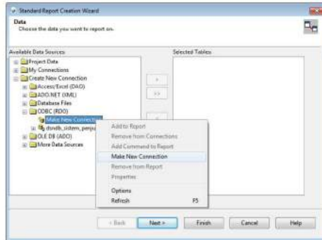
Gambar 8.8 Membuat Koneksi
