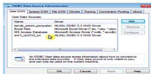
Gambar 4.20 ODBC Baru
