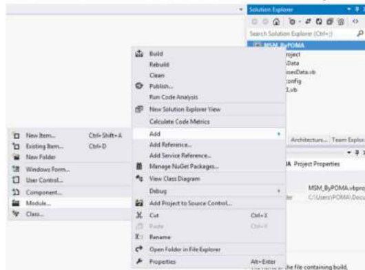
Gambar 5.11 ModulKoneksi
