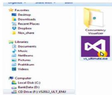
Gambar 4.1 Shortcut VB_2012
