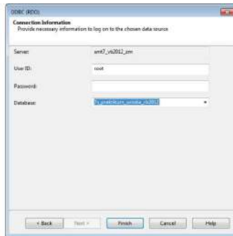
Gambar 8.10 Memilih Database
