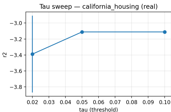
(d) California Housing (real)
