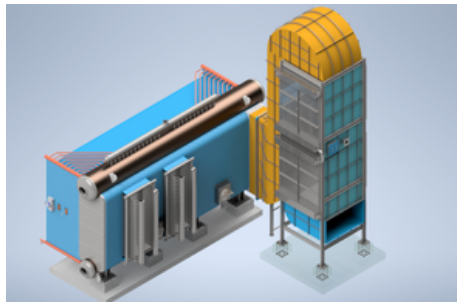
Рендер двухбарабанного парового котла
