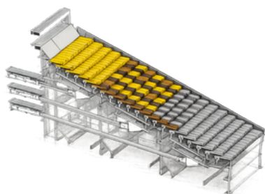
Концепция колосниковой системы сжигания
