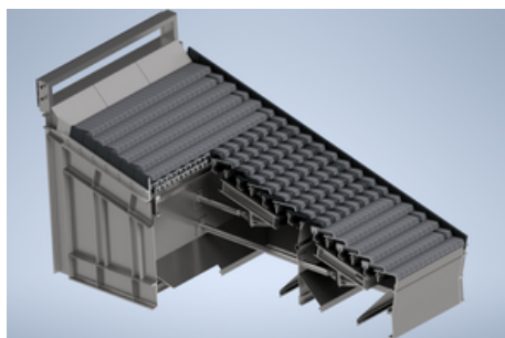
Рендер колосниковой системы сжигания
