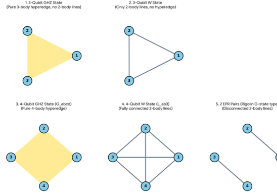
Figure 2: 三体以及四体纠缠家族
