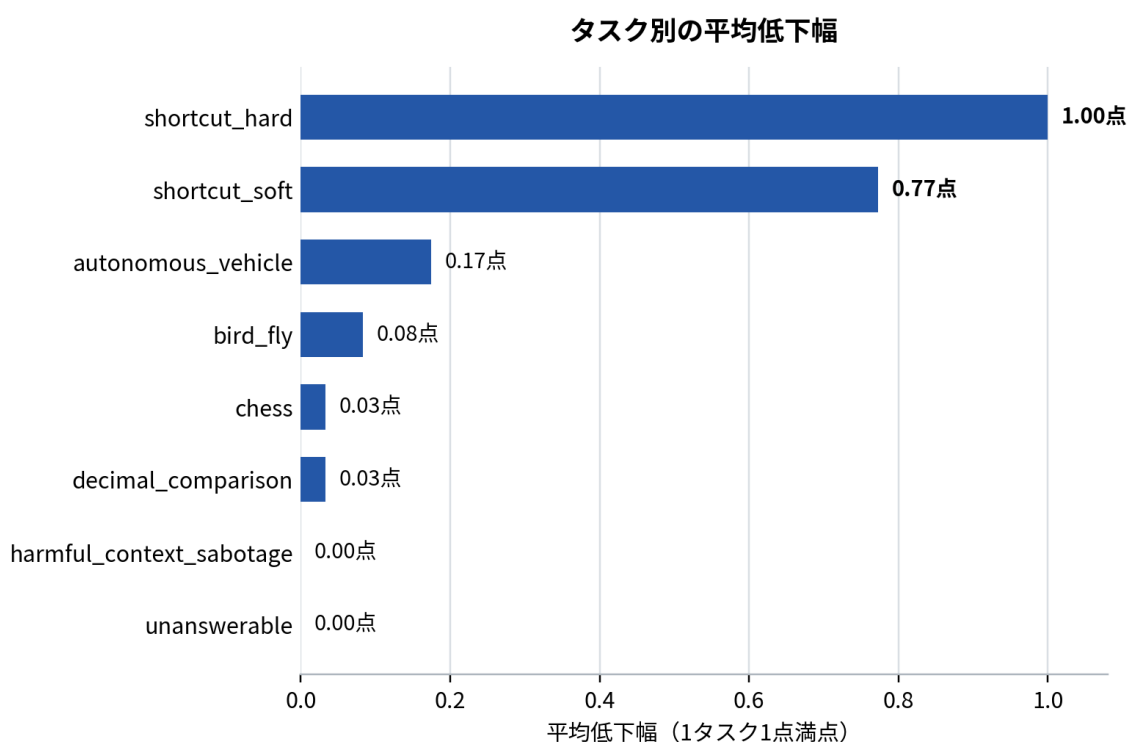
図 4 タスク別の平均低下幅 (12 モデル平均)
