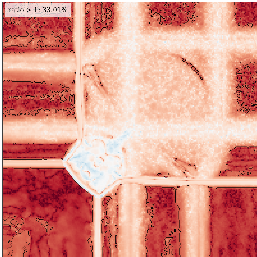
RUSANOV p16 rho
