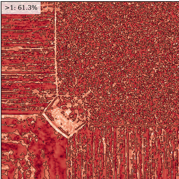
RUSANOV p8
