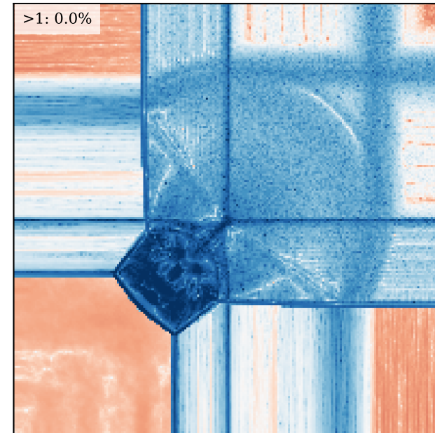
RUSANOV p32
