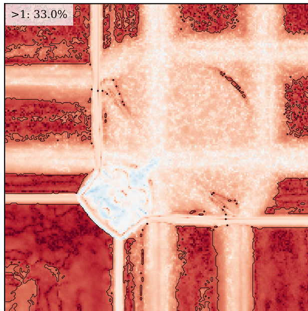
RUSANOV p16
