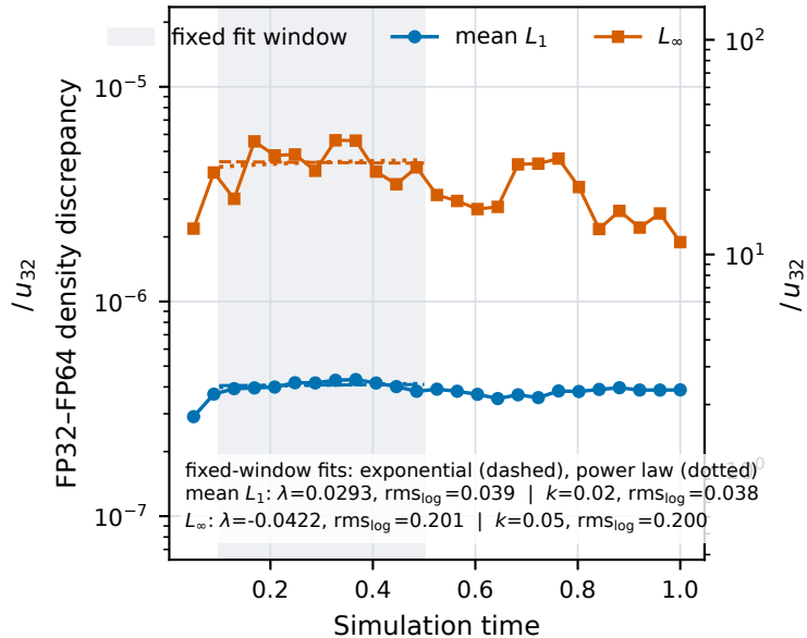
(b) Orszag-Tang
