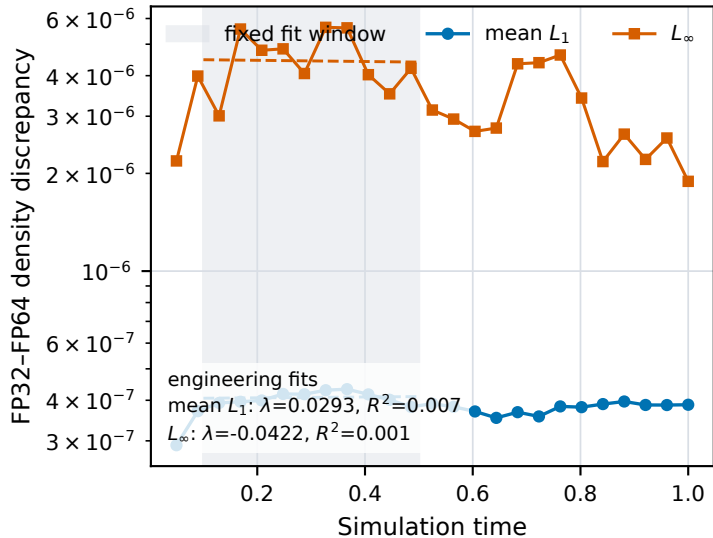
(b) Orszag-Tang
