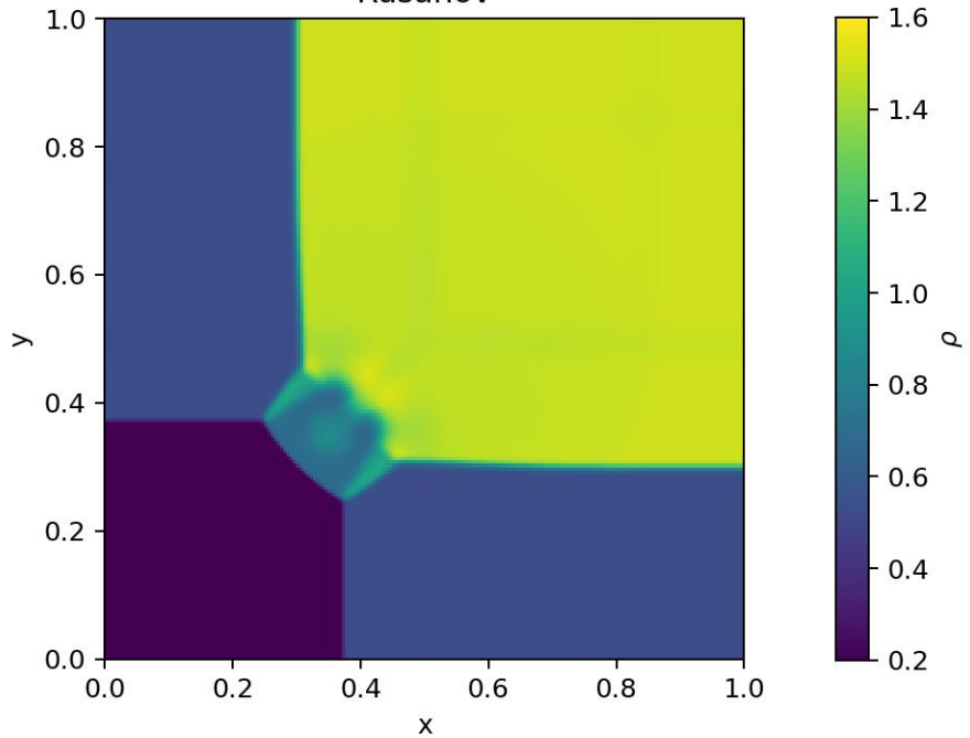
Rusanov
