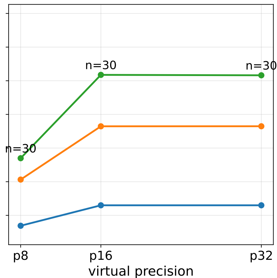
RUSANOV
