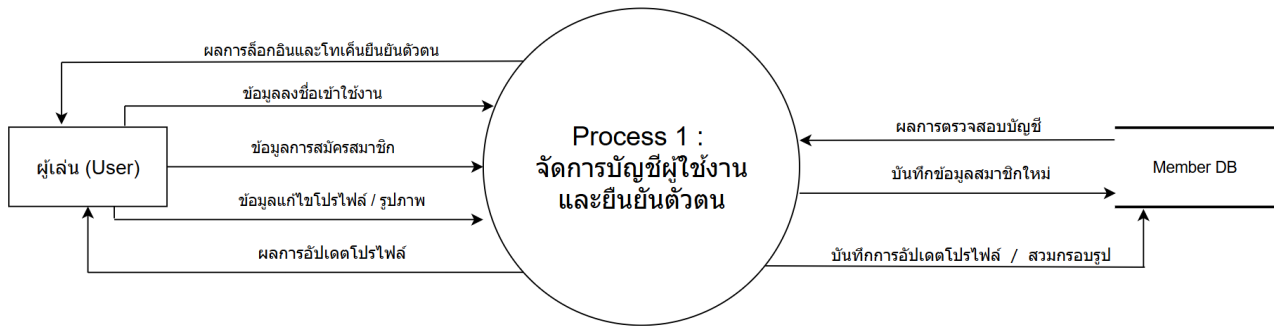
ภาพที่ 4 แผนภาพกระแสข้อมูลระดับ 1 (Process 1: จัดการบัญชีผู้ใช้งานและยืนยันตัวตน)
