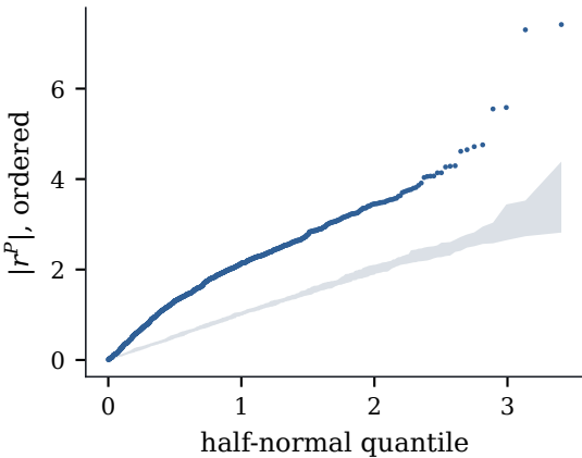
(a) binomial
