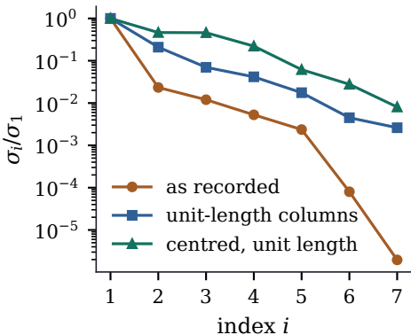
(a) singular values
