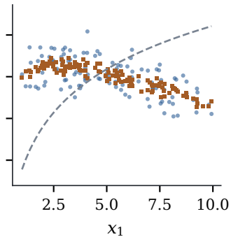
(b) x_2 \approx \sqrt{x_1}
