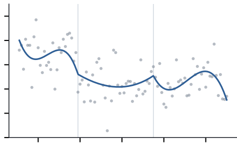
(d) cubic spline: 6 parameters
