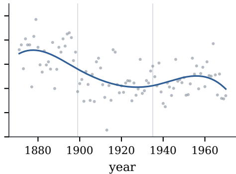
(d) cubic spline: 6 parameters
