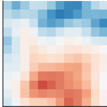
(d) kriging
