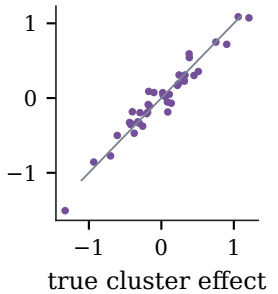
(d) random intercept
