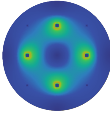
Fig. 5: Volumenstromverteilung auf der 1. Generation des Sensorlayouts
