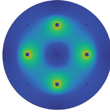
Fig. 5: Volumenstromverteilung auf der 1. Generation des Sensorlayouts
