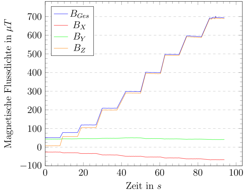
Graph 3: Gemessenes Magnetfeldkomponenten mit einem iPad-Magnetometer
