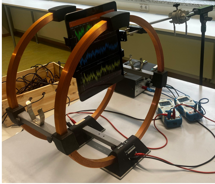
Fig. 7: Beispielhafter Versuchsaufbau mit iPad
