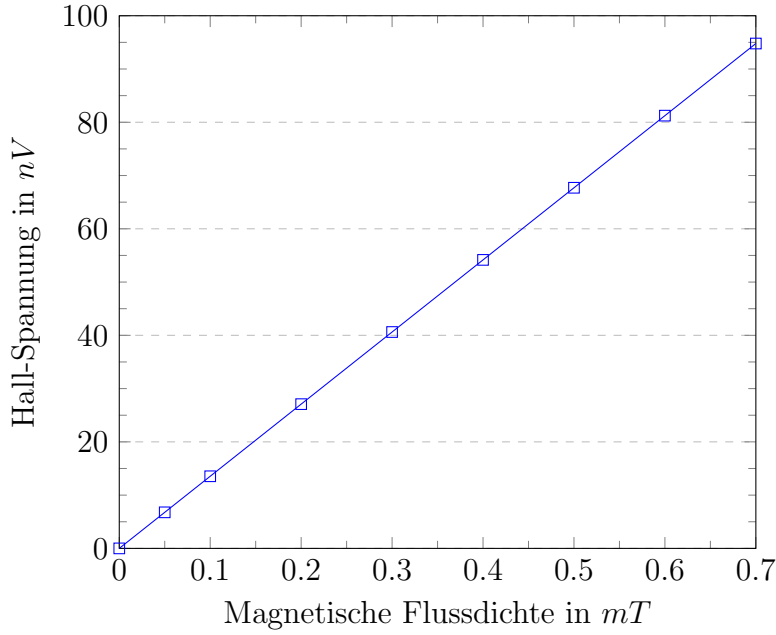
Graph 1: Hall-Spannung in der ersten Generation des Layouts
