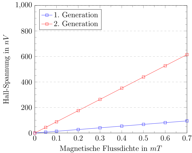
Graph 2: Hall-Spannung in der zweiten Generation des Layouts im Vergleich zur ersten Generation
