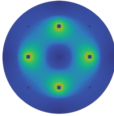
Fig. 5: Volumenstromverteilung in der 1. Generation des Sensorlayouts
